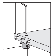
Piedino regolabile / Adjustable foot
