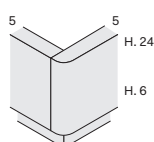
Particolare dell'unione tra longone e pediera Detail of join between side rail and footboard
