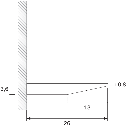
Senza schiena No back panel
