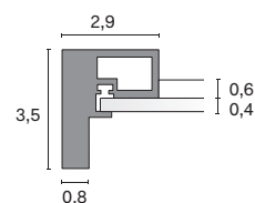
Sezione con cuoio e specchio / Cross-section with leather and mirror
