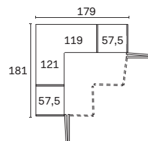
moduli angolo PANORAMA / PANORAMA corner modules
